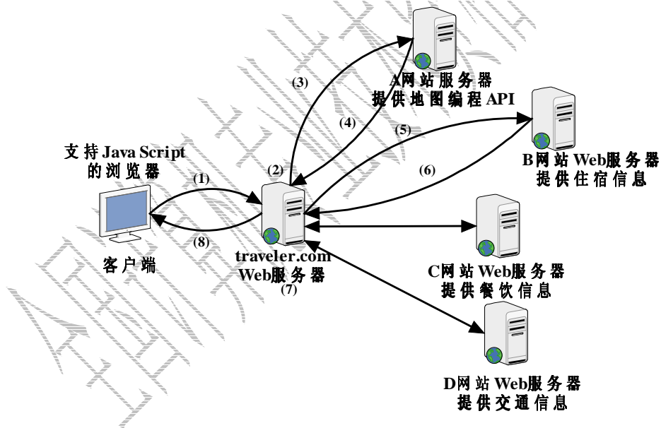
图 5-1 Mashup 流程示意图
